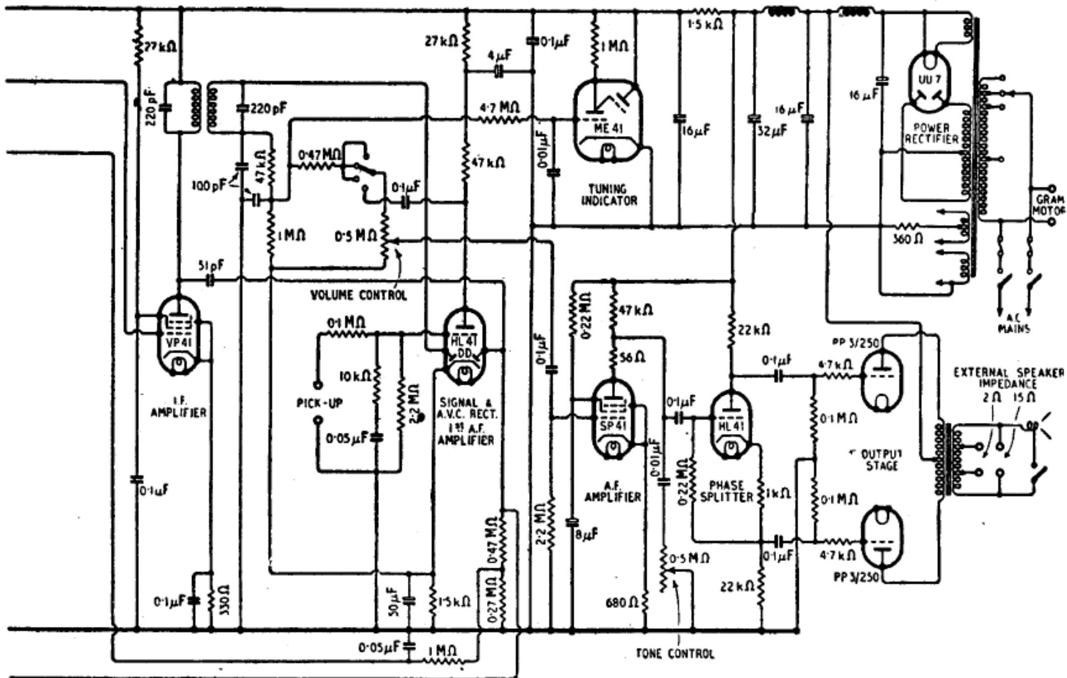
Parte MF e BF della supereterodina R.G.D. 1046 G.
